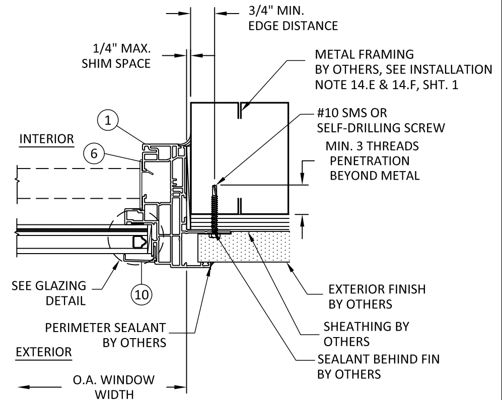
K 5 HORIZONTAL SECTION JAMB - METAL STUDS J-CHANNEL/NAIL FIN
